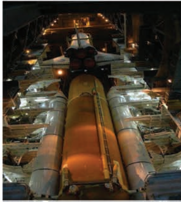
الشكل (٥) ربط المكوك الفضائي بصاروخي الإطلاق
